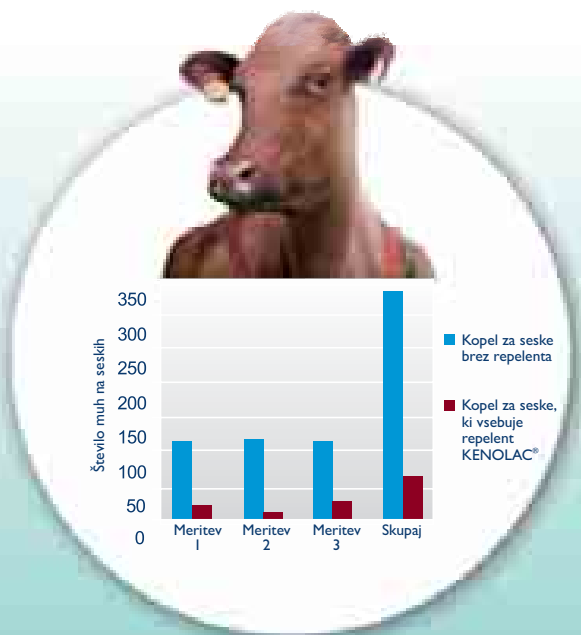
Grafikon: rezultati testiranja repelentne aktivnosti KENOLAC®-a
